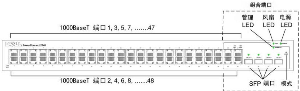
图 2-7. PowerConnect 2748 前面板
